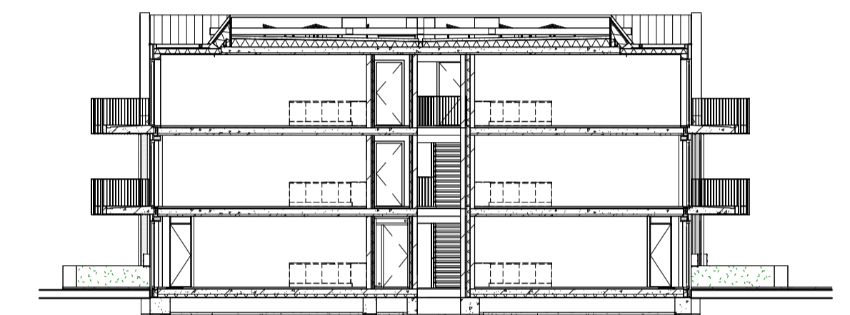
Doorsnede A-A
